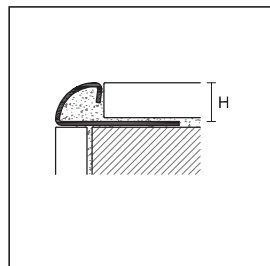
RIL/10 acier inox AISI 304 DIN 1.4301
