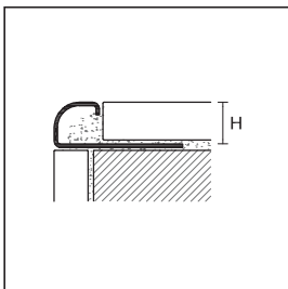
RIN/10 acier inox AISI 304 - DIN 1.4301
