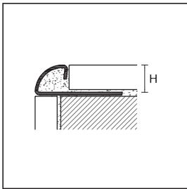
RKN/10 laiton chromé
